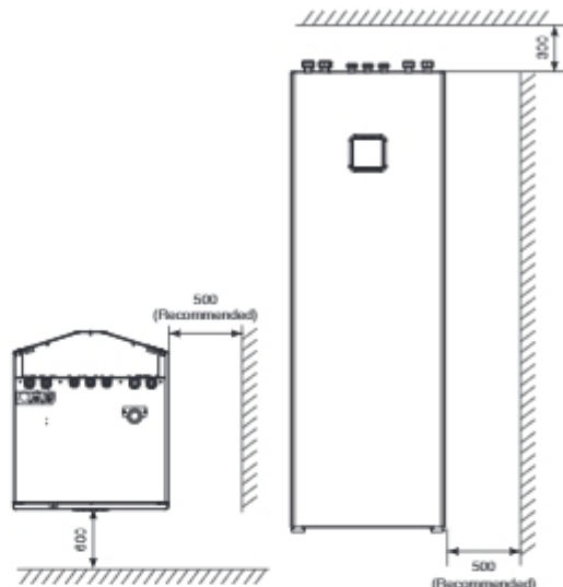
Minimální servisní prostor (jednotka: mm)
