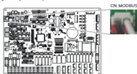
Vnitřní DPS
