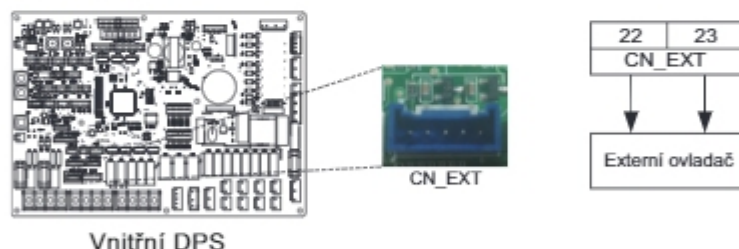
Příklad instalace #1
