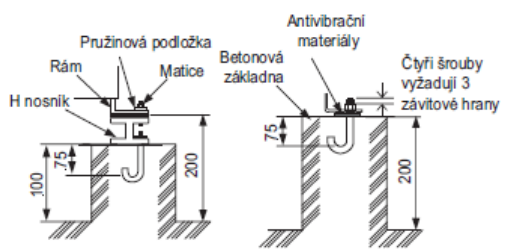
Způsob provedení základového šroubu
