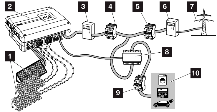
Fig. 2: Instalación fotovoltaica con sensor de corriente
