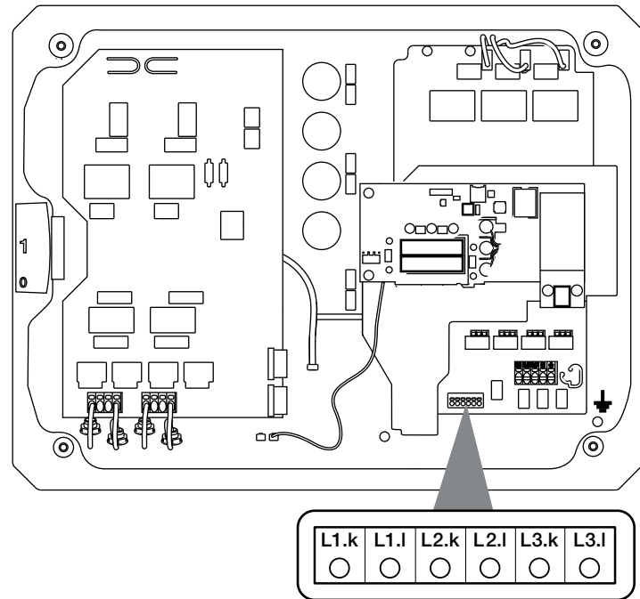
Fig. 6: Ligação do sensor de corrente ao inversor
