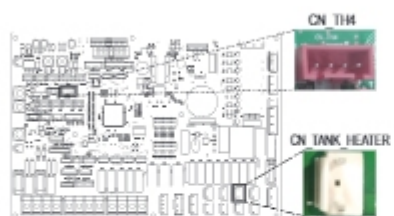
Vnitřní DPS
