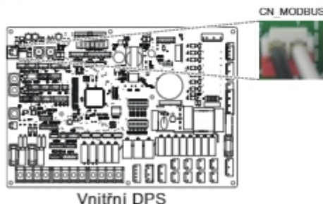
Vnitřní DPS
