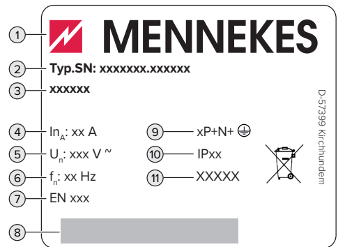
Obr. 1: Typový štítek (vzor)
