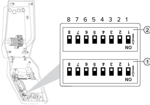
Şek. 11: DIP şalteri (teslimattaki durum)
