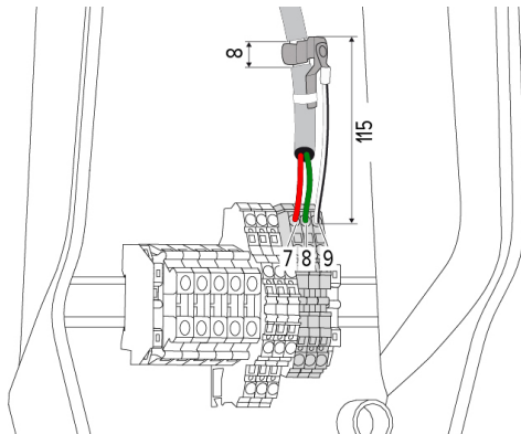
Fig. 10: Tilslutning dataledning [mm]
