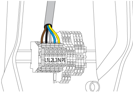
Abb. 8: Anschluss Spannungsversorgung
