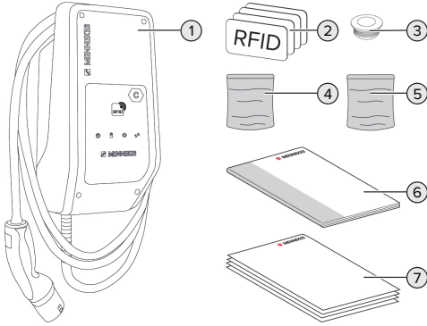
Kuva 2: Toimituksen laajuus
