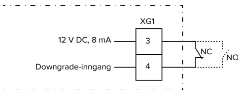
Fig. 13: Prinsipielt koblingsskjema: tilkobling av en ekstern bryterkontakt (standardinnstilling: NC)
