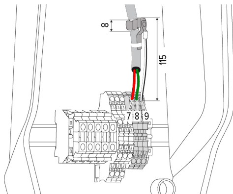
Εικ. 10: Σύνδεση καλωδίου δεδομένων [mm]
