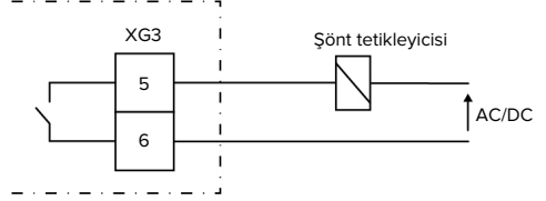
Şek. 9: Prensipsel devre şeması: Harici bir şönt tetikleyicisinin bağlanması
