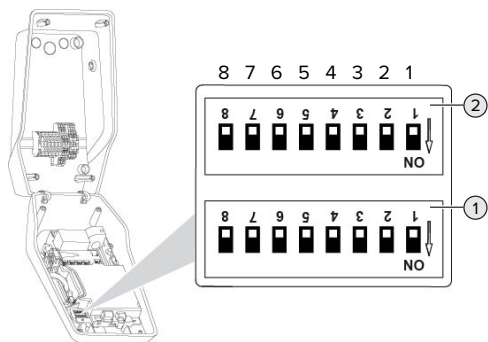
Fig. 11: Interruptores DIP (estado de entrega)
