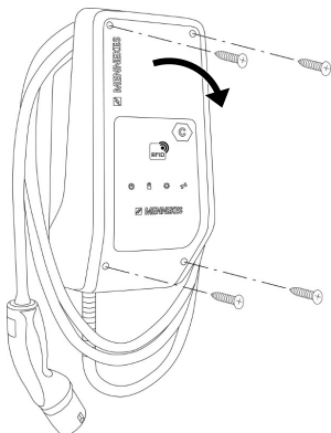
Obr. 5: Otevření výrobku
