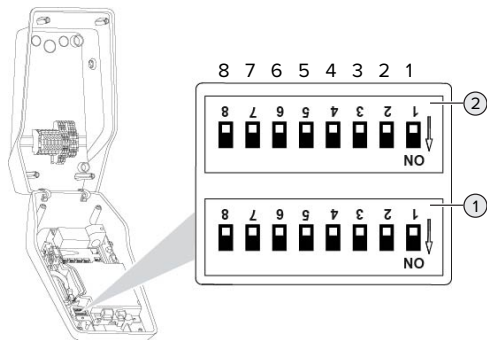
Ilustr. 11: Przełącznik DIP (stan dostawy)
