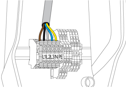
Kuva 8: Jännitesyötön liitäntä
