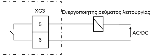
Εικ. 9: Διάγραμμα συνδεσμολογίας: Σύνδεση εξωτερικού ενεργοποιητή ρεύματος λειτουργίας
