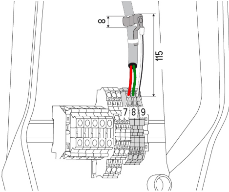
Şek. 10: Veri hattı bağlantısı [mm]
