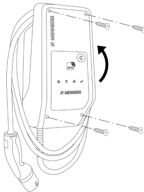
Fig. 16: Fechar o produto
