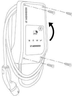
Kuva 16: Tuotteen sulkeminen
