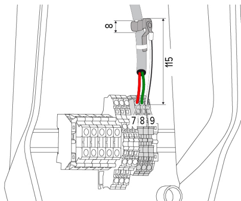
Ilustr. 10: Przyłącze przewodu danych [mm]
