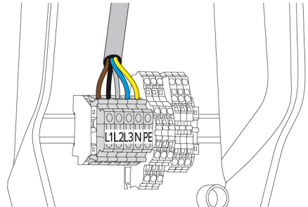
Pav. 8: Aprūpinimo įtampos jungtis
