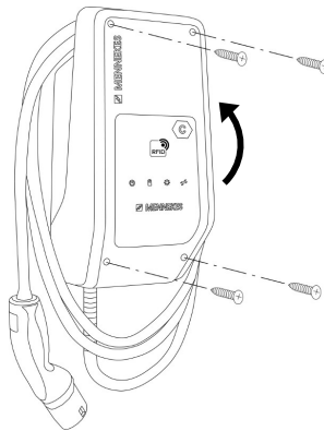
Pav. 16: Gaminį uždaryti
