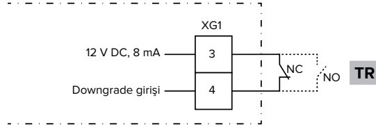
Şek. 13: Prensipsel devre şeması: Harici bir şalter kontağının bağlanması (standart ayar: NC)
