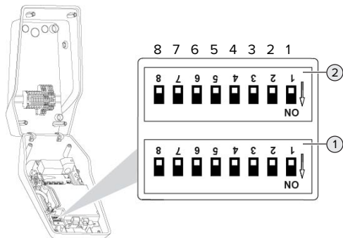
Fig. 11: DIP-kontakter (udleveringstilstand)
