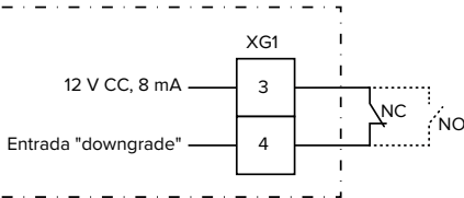
Fig. 13: Esquema de princípio: ligação de um contacto de comutação externo (configuração padrão: NF)
