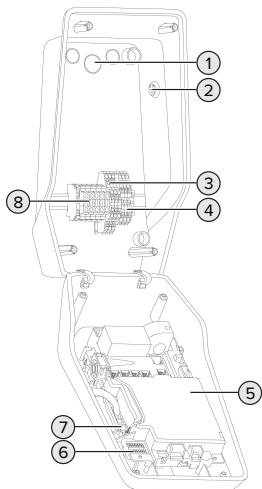
Obr. 4: Pohled dovnitř
