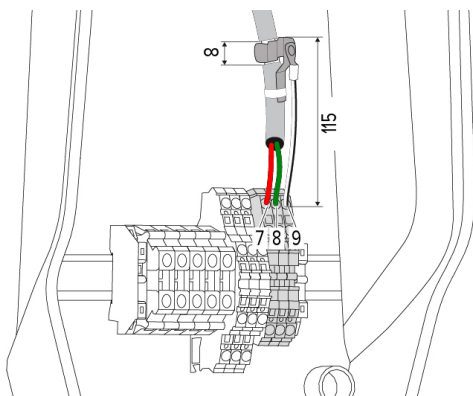
sl. 10: Priključek podatkovnega voda [mm]
