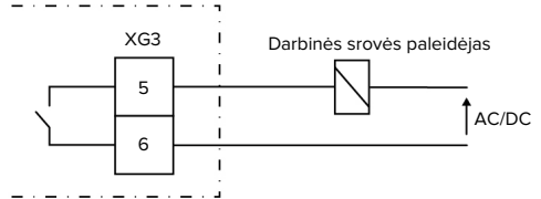
Pav. 9: Esminis jungimo paveikslėlis: išorinio darbinės srovės paleidėjo prijungimas
