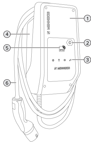
Fig. 3: Vista exterior
