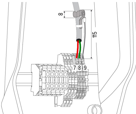
Kuva 10: Tietojohdon liitäntä [mm]
