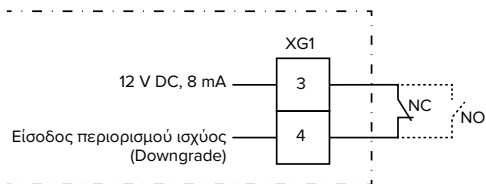
Εικ. 13: Διάγραμμα συνδεσμολογίας: Σύνδεση εξωτερικής επαφής μεταγωγής (βασική ρύθμιση: NC)
