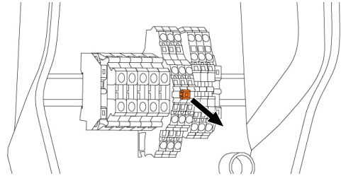
Kuva 12: Hyppyjohtimen poistaminen
