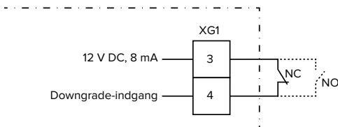
Fig. 13: Principskema: tilslutning af en ekstern omskifterkontakt (standardindstilling: NC)
