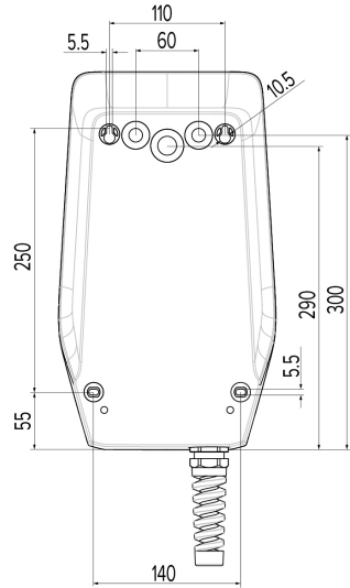
Εικ. 6: Διαστάσεις διάτρησης [mm]
