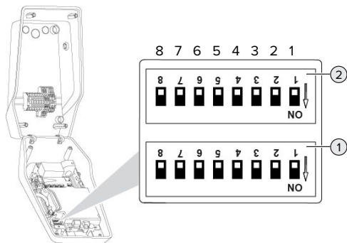
Obr. 11: DIP přepínače (stav při dodání)
