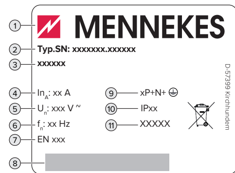
Pav. 1: Tipų skydas (pavyzdys)
