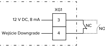
Ilustr. 13: Schemat blokowy: podłączenie zewnętrznego styku przełączającego (ustawienie standardowe: NC)
