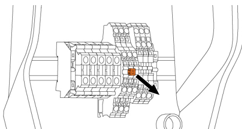
Fig. 12: Tag kortslutningstråden ud
