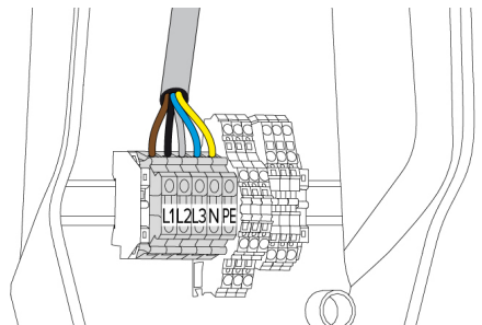
Fig. 8: Tilslutning strømforsyning
