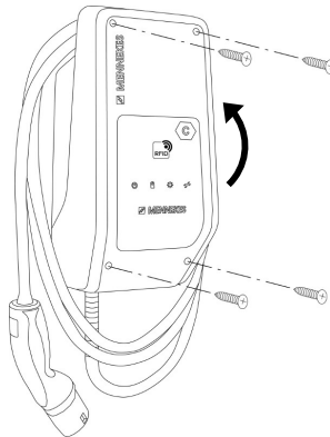
Abb. 16: Produkt schließen
