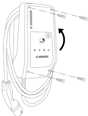
Εικ. 16: Κλείσιμο του προϊόντος
