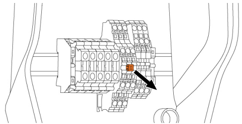
Pav. 12: Tiltą išimti
