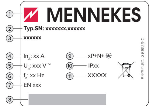
Kuva 1: Tyyppikilpi (malli)
