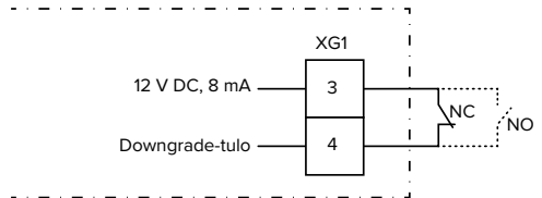
Kuva 13: Periaatekytkentäkaavio: ulkoisen kytkentäkontaktin liitäntä (vakioasetus: NC)
