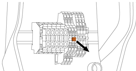
Ilustr. 12: Wyjmowanie mostka
