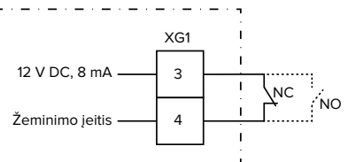
Pav. 13: Esminis jungimo paveikslėlis: išorinio jungimo kontakto prijungimas (standartinis nustatymas: NC)
