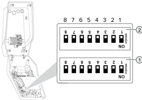
Pav. 11: DIP jungiklis (būsena pristatymo metu)
