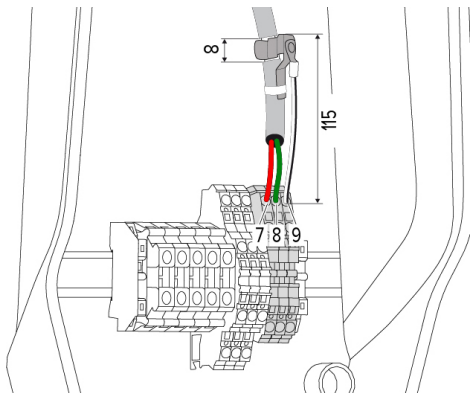
Obr. 10: Přípojka datového kabelu [mm]
