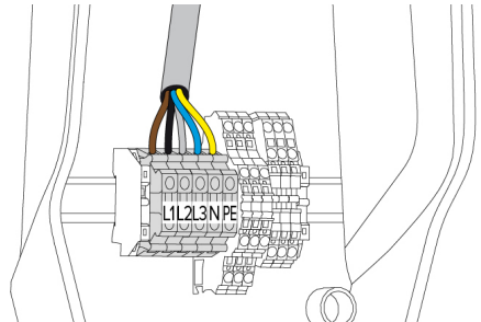
Obr. 8: Připojení zdroje napětí
