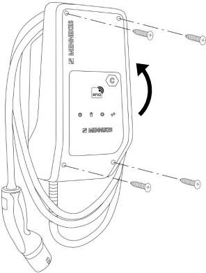
Şek. 16: Ürünün kapatılması
