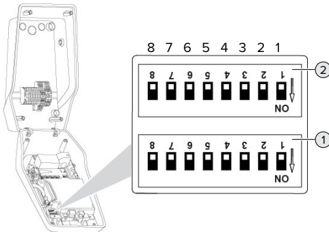
Εικ. 11: Διακόπτες DIP (κατάσταση κατά την πα- ράδοση)
