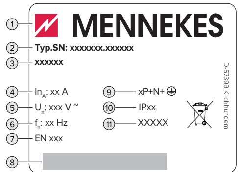
Fig. 1: Typeskilt (eksempel)
