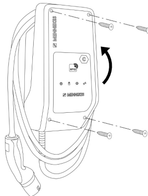
Obr. 16: Zavření výrobku
