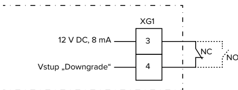
Obr. 13: Základní schéma: Připojení externího spínacího kontaktu (standardní nastavení: NC)
