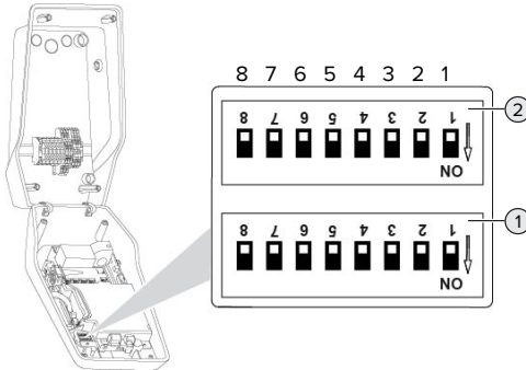
Kuva 11: DIP-kytkin (toimitustila)
