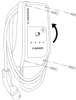
Fig. 16: Lukke produktet
