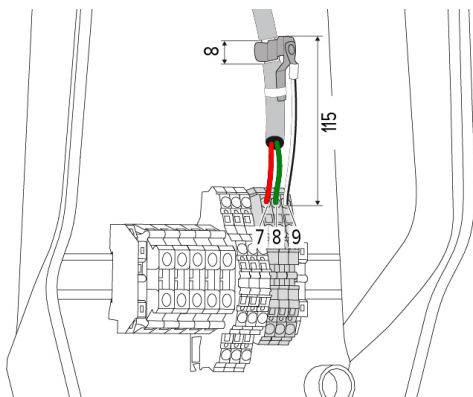
Pav. 10: Jungtis duomenų linija [mm]
