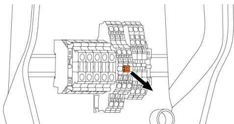
Εικ. 12: Αφαίρεση γέφυρας
